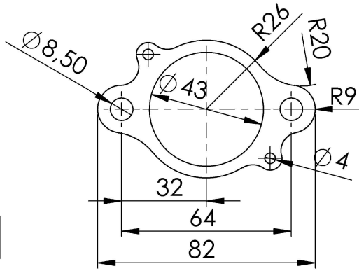
4 S.S. Flange Cod."205670"
